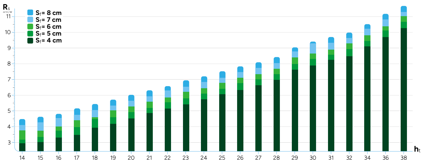
Diagramma delle resistenze termiche ottenibili al variare dello spessore S_t dell'altezza strutturale H_t
